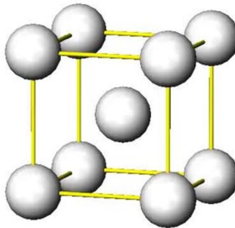
Cubique centré
